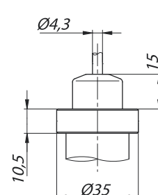
Кабельный ввод
