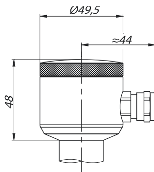
Компактный полевой корпус
